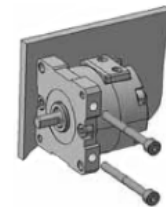
Verwendung der Durchgangsbohrungen in der Platte
