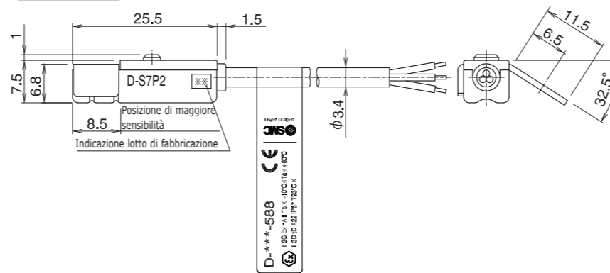
D-S7P□DPC-588
