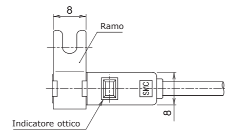
D-S7P2-588
