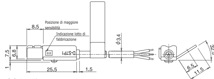
D-S7P1-588
