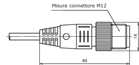
D-S7P□DPC-588
