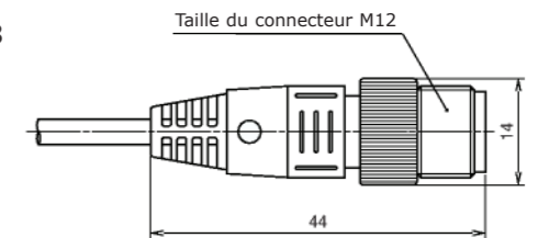
D-S9P□DPC-588
