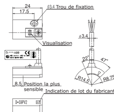
D-S9PV2-588
