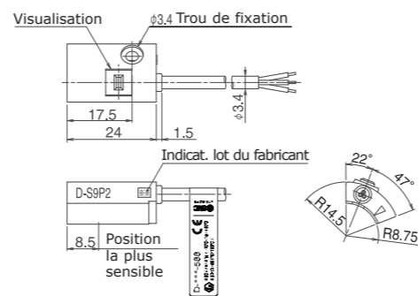
D-S9P2-588
