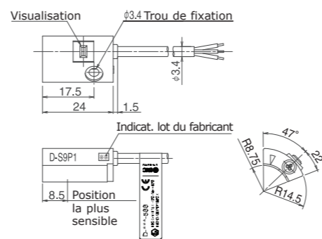
D-S9P1-588
