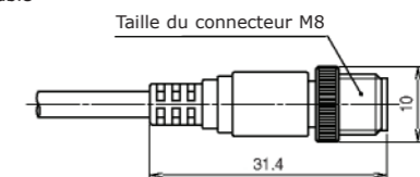
D-S9P□PC-588
