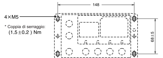
Dimensioni della scontornatura per il montaggio (Tolleranza: 0.2)
