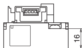
Cubierta retirada (Tolerancia ± 0.2 mm)
