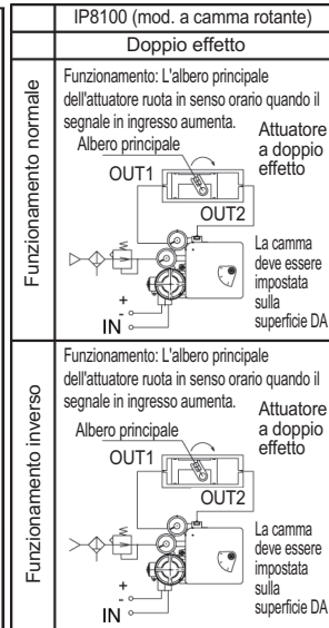
FIG. 5 Funzionamento diretto/inverso
