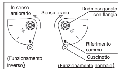
Fig.4 Esempio di collegamento della camma
