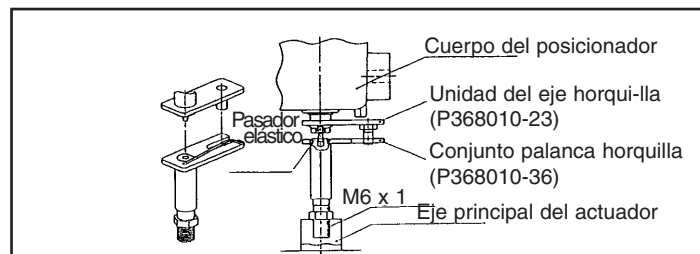
Fig.8 Montaje de la palanca de retroalimentación
