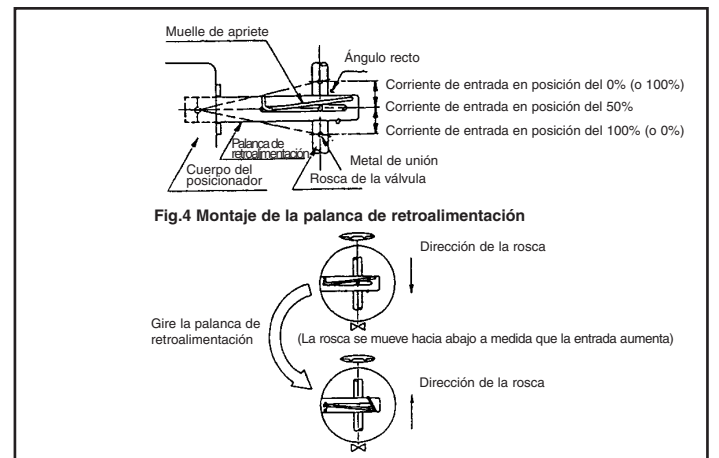
Fig.5 Posición de uso para la palanca de retroalimentación
