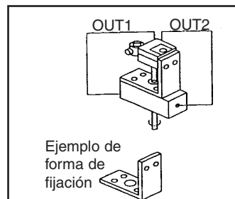
Fig.6 Ejemplo de montaje mediante el tornillo lateral del posicionador
