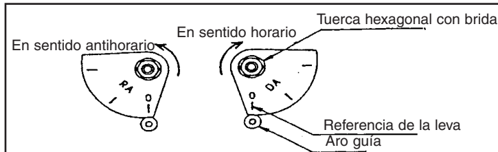
Fig.9 Ejemplo de montaje de la leva
