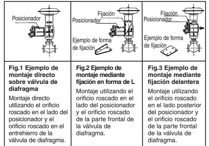
Fig.1 Ejemplo de montaje directo sobre válvula de diafragma Montaje directo utilizando el orificio roscado en el lado del posicionador y el orificio roscado en el entrehierro de la válvula de diafragma.
