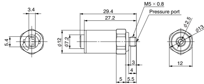
PSE53□-R06 R07
