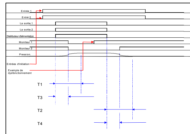
Voir le tableau relatif aux temps de réponse du distributeur et du détecteur T1, T2, T3, T4
