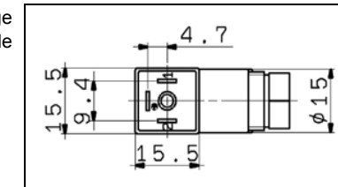
Borniers du connecteur Vue du côté du distributeur
